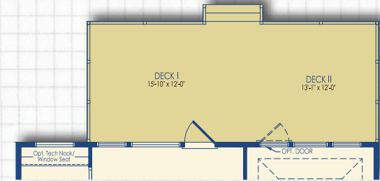
Optional Decks I & II
