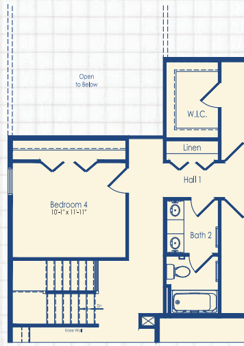
Optional Bedroom 4
