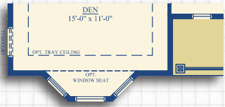
Optional Den Elevation B and C
