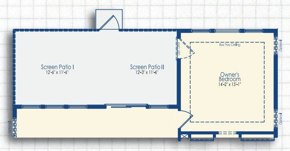
Optional Screen Patio I & II
