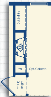
Optional Inset Fireplace
