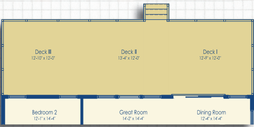
Optional Deck I, II, & III
